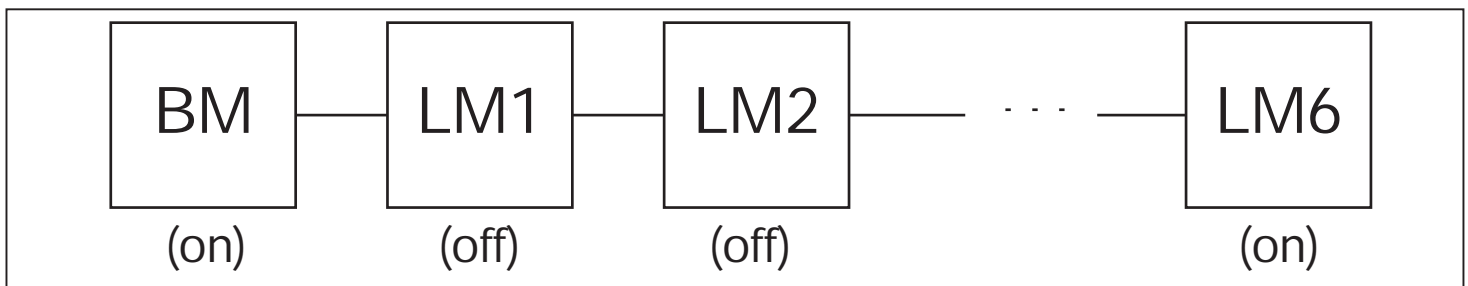
BM ... Basismodul ES5403 (oder auch Kompakt-Wandler ES5400) LM1 – LM6 ... Lesemodul 1 bis Lesemodul 6
