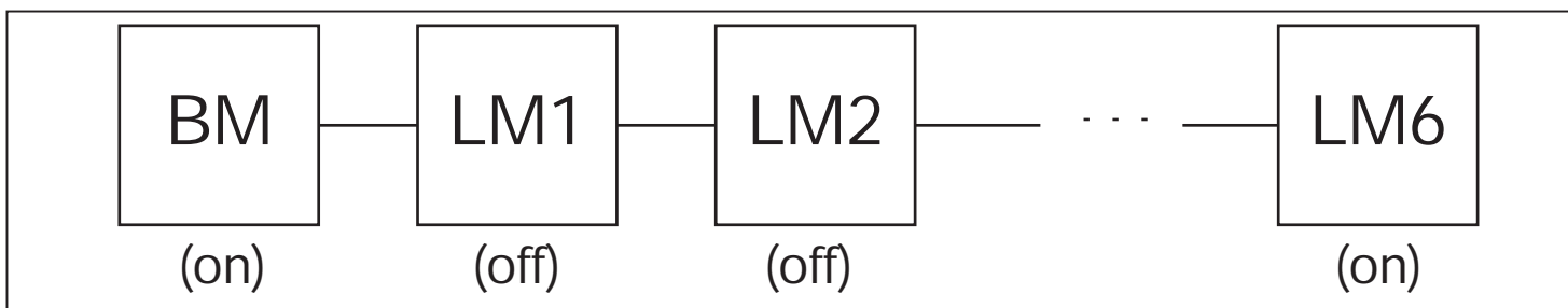
BM ... Module de base ES5403 (ou également lecteur mural compact ES5400) LM1 – LM6 ... Module de lecture 1 à module de lecture 6
